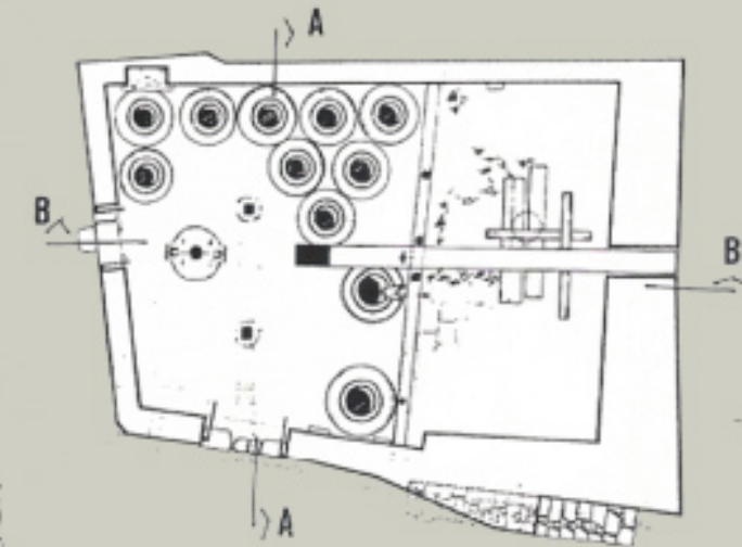
Κάτοψη Ληνού
