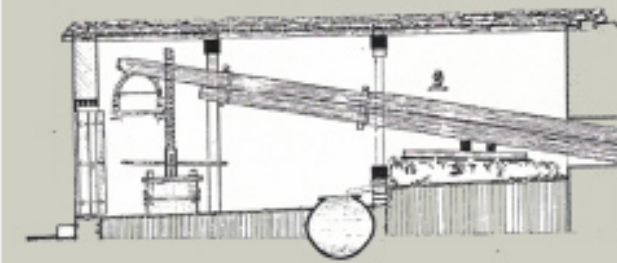
Τομή ΑΑ' Ληνού
